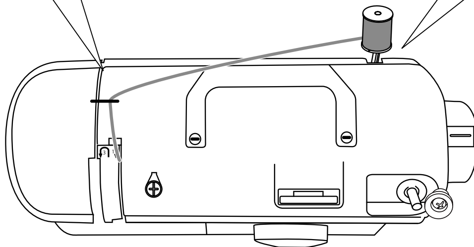
< ミシン上面図 >
