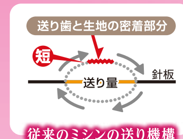
従来のミシンの送り機構
